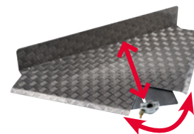
Plateau d'angle réglable 0 à 90° Largeur : 800 mm ou 1000 mm selon le modèle
