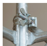
Fixation des diagonales
