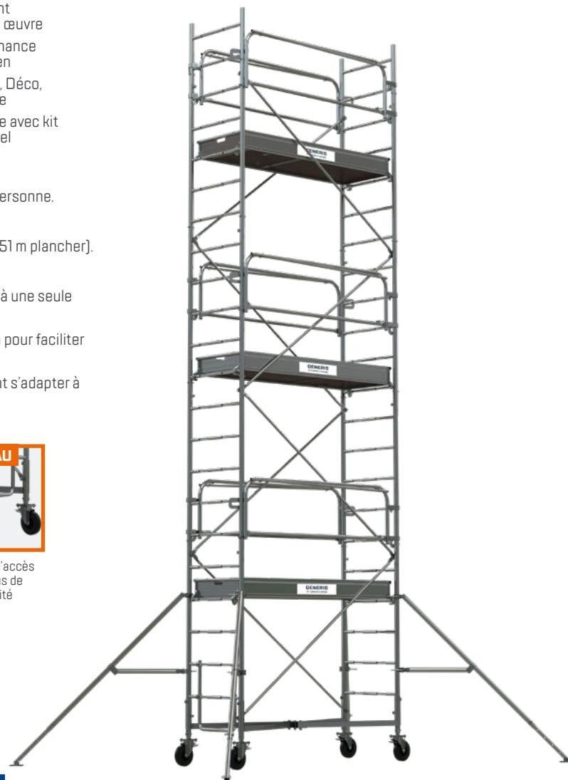
GENERIS 750 5,80 m plancher
