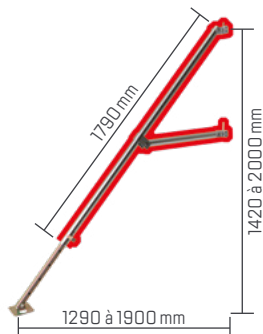
Stabilisateur S1
