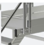
Liaison plan de montée / plate-forme très résistante
