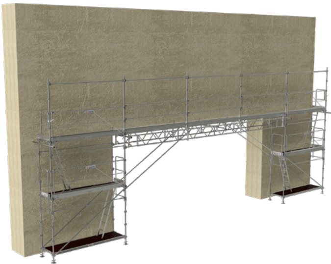
Pont 6 m : 2 poutres aluminium de 5,10 m en vis à vis
