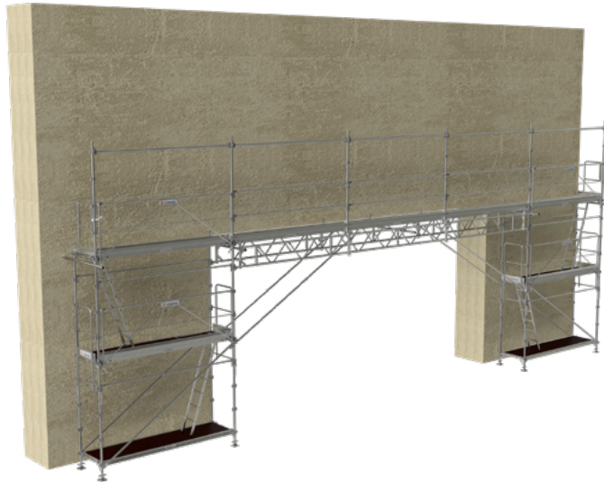
A Pont 6 m : 2 poutres aluminium de 5,10 m en vis à vis
