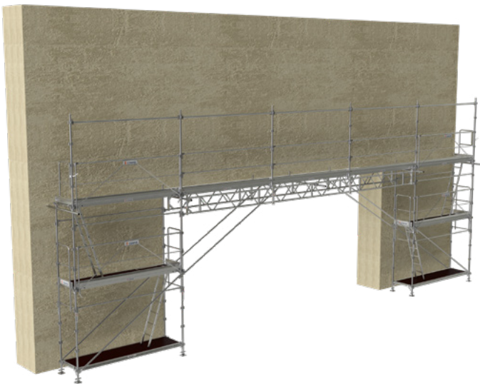
Pont 6 m : 2 poutres aluminium de 5,10 m en vis à vis
