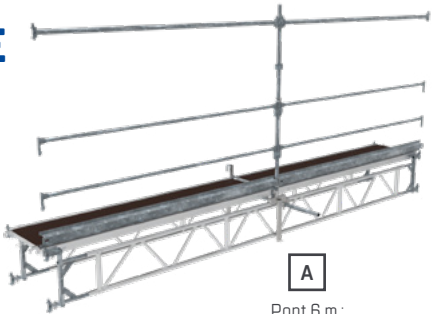
Pont 6 m : 2 poutres aluminium de 5,10 m en vis à vis
