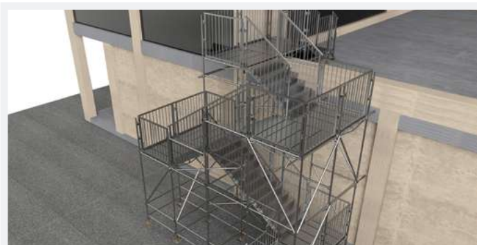
Escalier quart et demi tournant avec palier en 2 ou 3 unités de passage permettant l'accès à une toiture terrasse. Cette configuration peut également être utilisée en sortie de secours.
