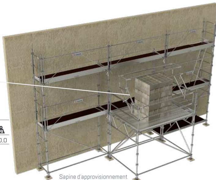
Sapine d'approvisionnement avec garde-corps basculant
