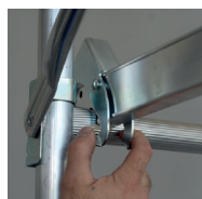
Système T-GRIP pour un montage et démontage en totale sécurité
